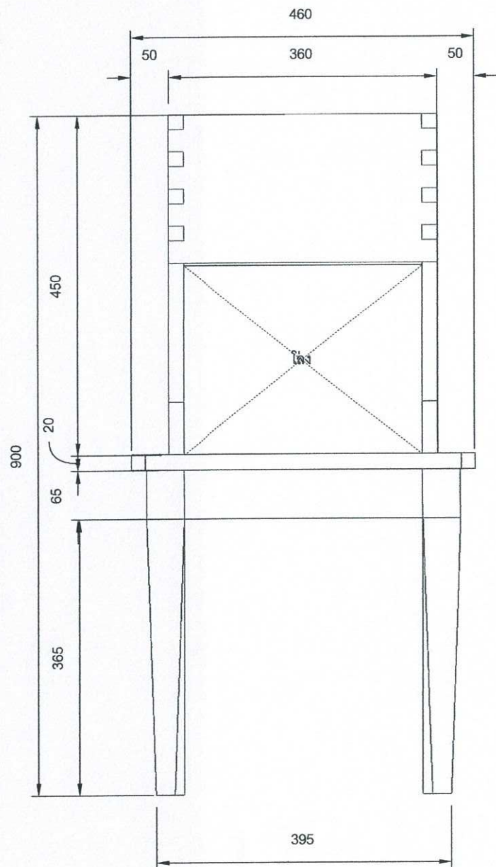
รูปด้านหน้า มาตราส่วน 1:5
