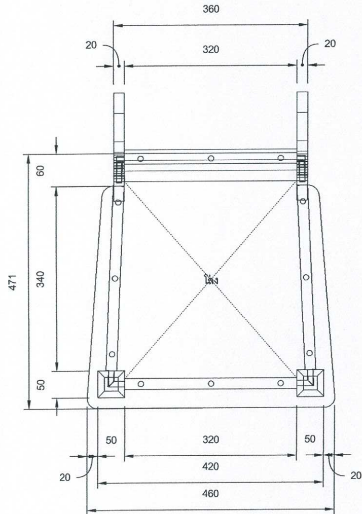
รูปตีนบน (ไม่มีพื้นทึบ) มาตราส่วน 1:5
