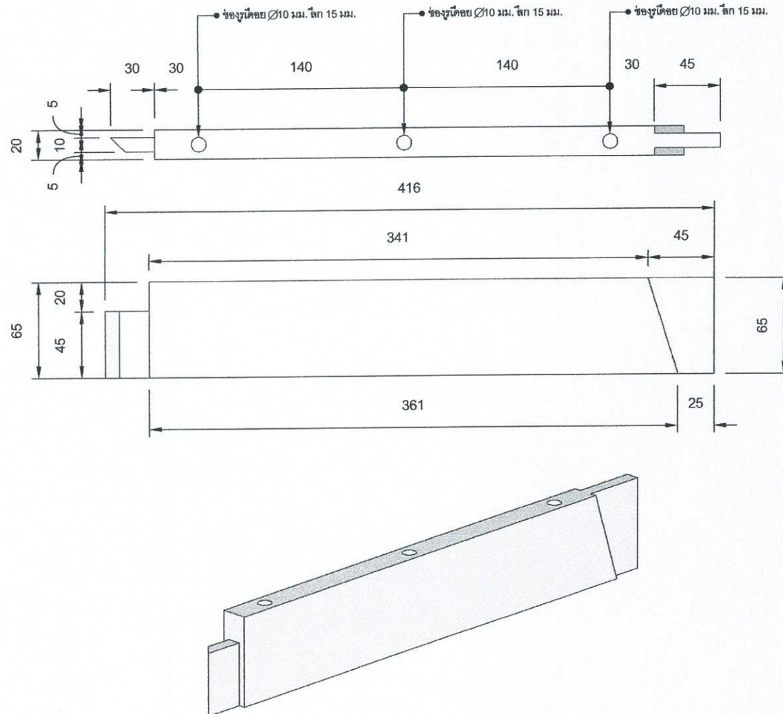
E1,E2 พนักรับพื้นนั่งข้าง มาตราส่วน 1:2.5
