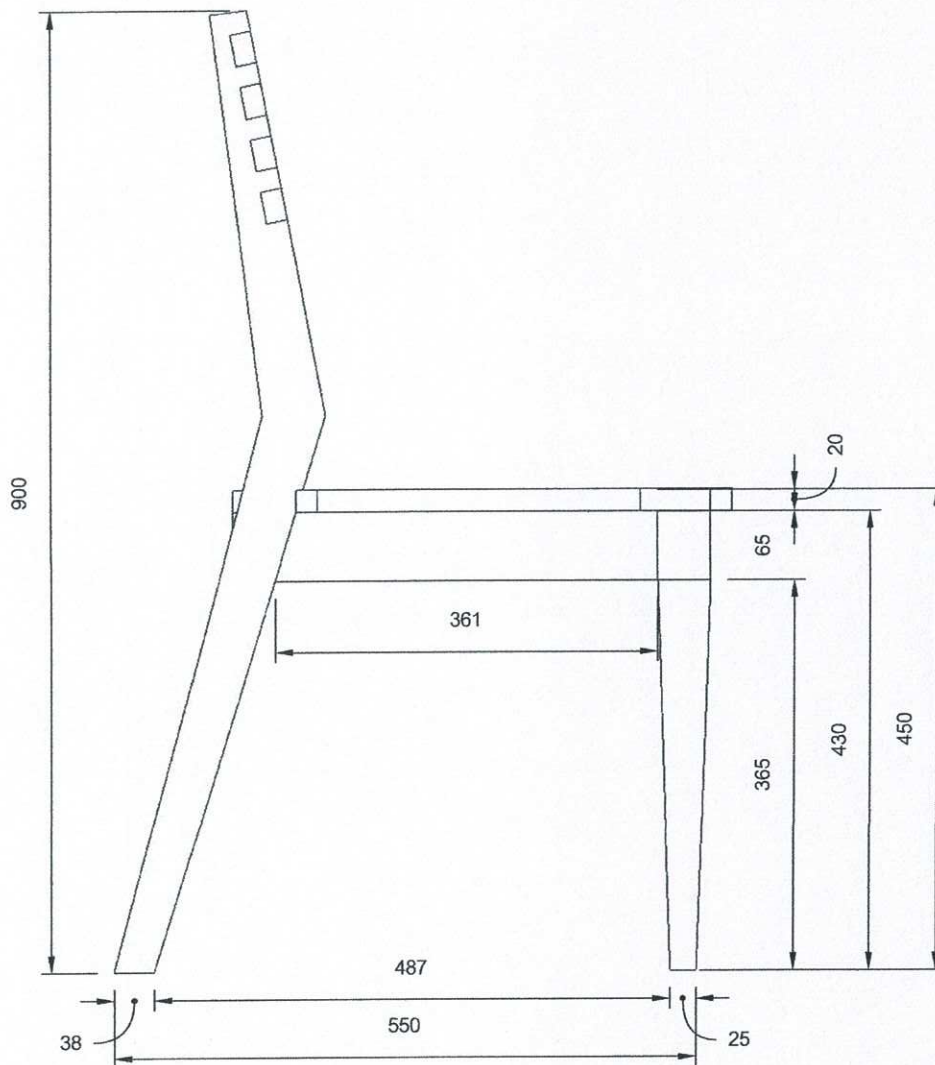
รูปด้านข้าง มาตราส่วน 1:5
