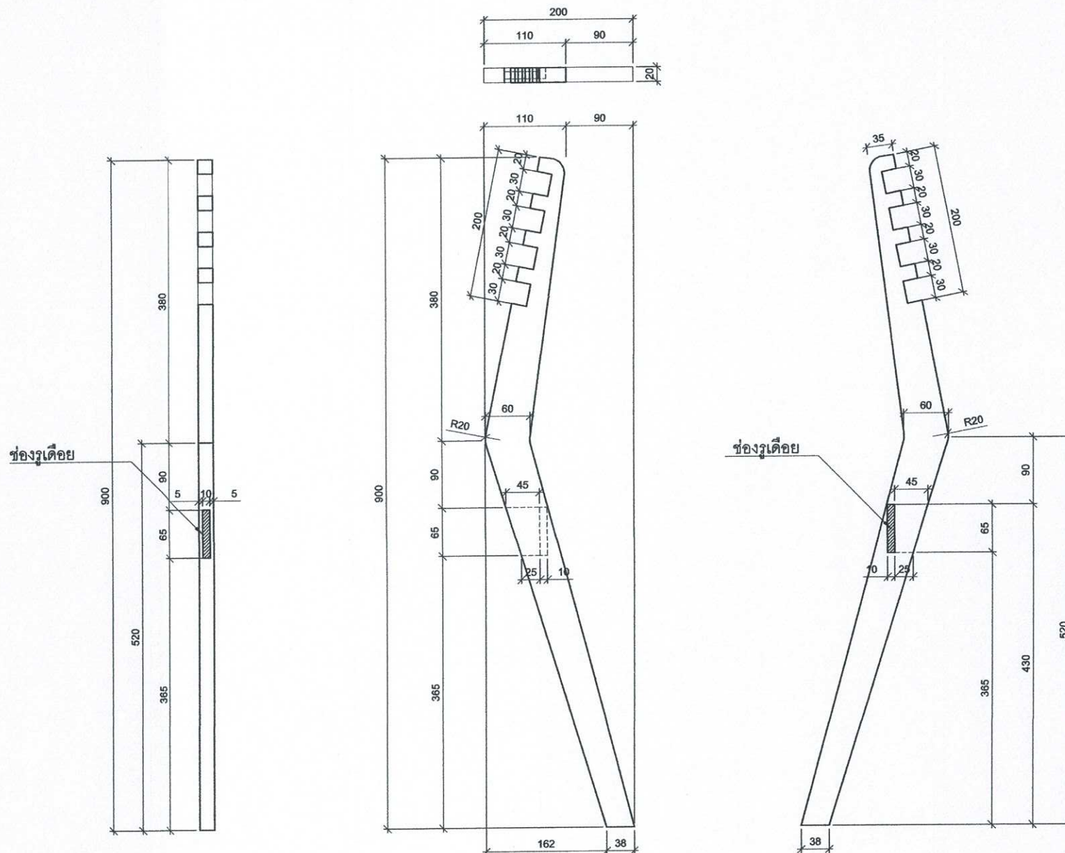
B1,B2 ขาเก้าอี้ด้านหลัง 1,2
